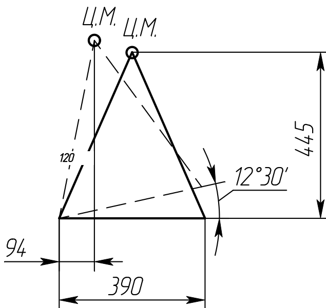
Рисунок 1- Схема устойчивости электронасосного агрегата типа 1ЦНСг60-198
